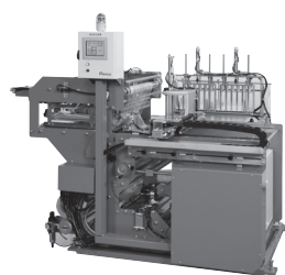
規格袋包装機 KH型
